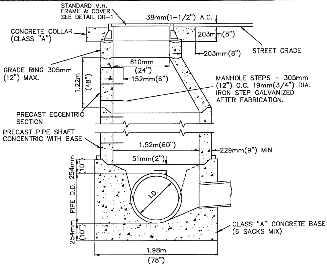
SECTION A-A
